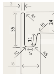
Z3 (RADIUS r2mm nebo r3mm)
