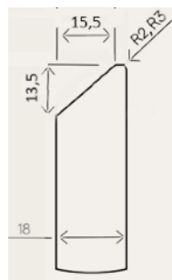
Z1 (RADIUS r2mm nebo r3mm)
