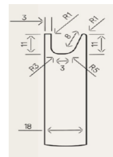
Z4 (RADIUS r2mm nebo r3mm)
